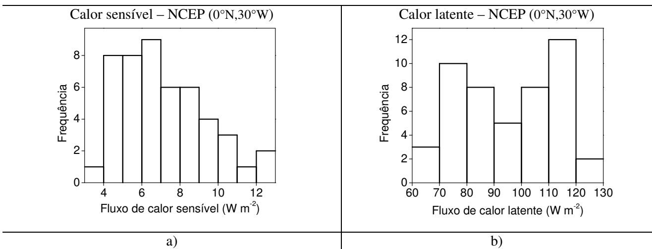
Figura 17: Histograma das médias diárias mensais dos fluxos verticais turbulentos de a) calor sensível e b) calor latente para o NCEP na localização 0°N e 30°W.
