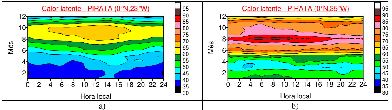
Figura 16: Evolução do fluxo vertical turbulento de calor latente calculado com os dados do projeto PIRATA, para as localizações a) 0°N e 23°W – B23W e b) 0°N e 35°W – B35W.
