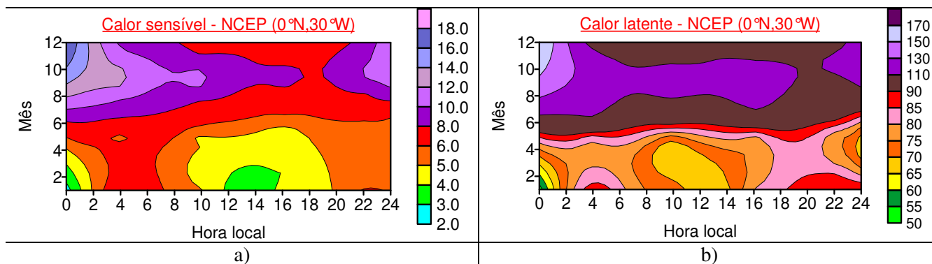
Figura 14: Evolução dos fluxos verticais turbulentos de a) calor sensível e b) calor latente para o NCEP na localização 0°N e 30°W.
