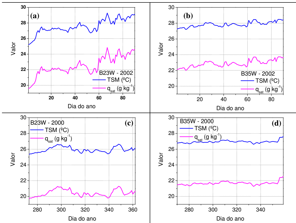
Figura 7: Temperatura da superfície do mar e a respectiva umidade específica de saturação calculada para esta temperatura, obtidas pelas duas Bóias PIRATA B23W e B35W, em dois períodos de tempo diferentes.
