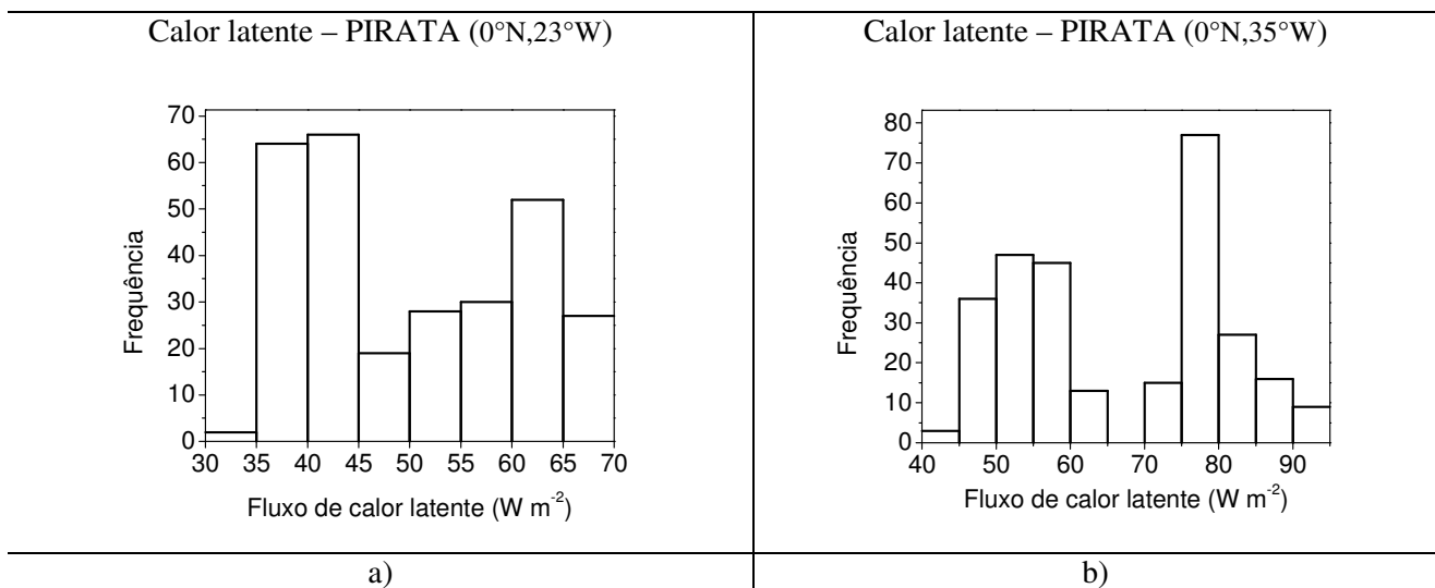
Figura 19: Histograma das médias diárias mensais do fluxo vertical turbulento de calor latente calculado com os dados do projeto PIRATA, para as localizações a) 0°N e 23°W – B23W e b) 0°N e 35°W – B35W.
