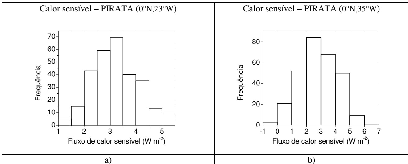
Figura 18: Histograma das médias diárias mensais do fluxo vertical turbulento de calor sensível calculado com os dados do projeto PIRATA, para as localizações a) 0°N e 23°W – B23W e b) 0°N e 35°W – B35W.
