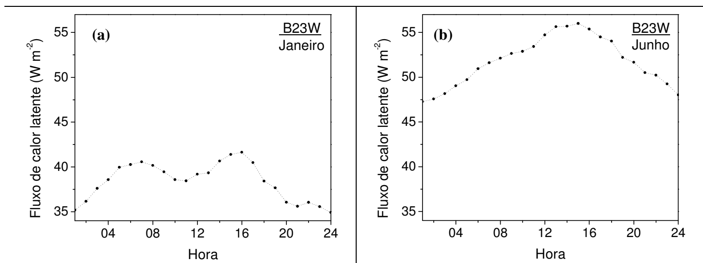
Figura 11: Médias horárias para os meses de janeiro e junho do fluxo turbulento vertical de calor latente estimado para a região da Bóia PIRATA B23W.
