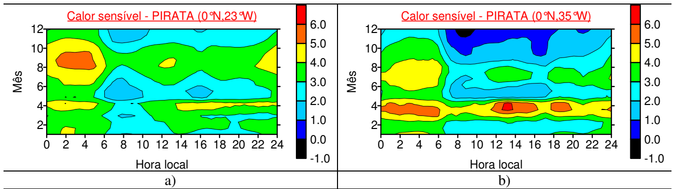
Figura 15: Evolução do fluxo vertical turbulento de calor sensível calculado com os dados do projeto PIRATA, para as localizações a) 0°N e 23°W – B23W e b) 0°N e 35°W – B35W.
