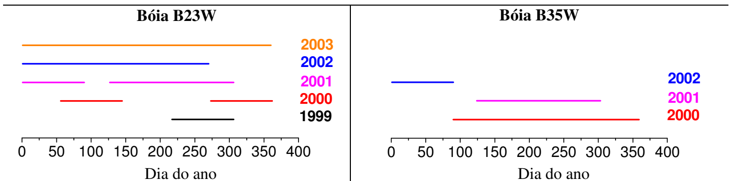
Figura 4: Série temporal dos dados de temperatura do ar e da superfície do mar, vento e umidade relativa distribuídos aos alunos do curso de Micrometeorologia.
