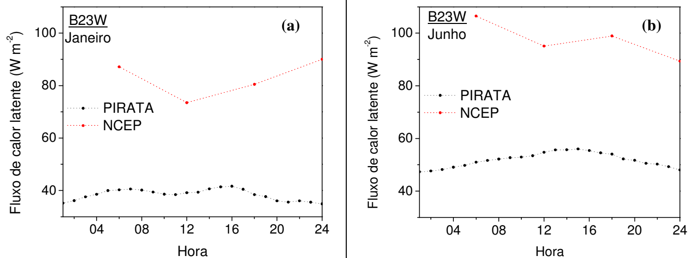
Figura 13: Médias horárias para os meses de janeiro e junho do fluxo turbulento vertical de calor latente estimado para a região da Bóia PIRATA B23W (pontos pretos) e para a região ( 0^{\circ}\text{N} , 30^{\circ}\text{W} ) dos dados de reanálise do NCEP.
