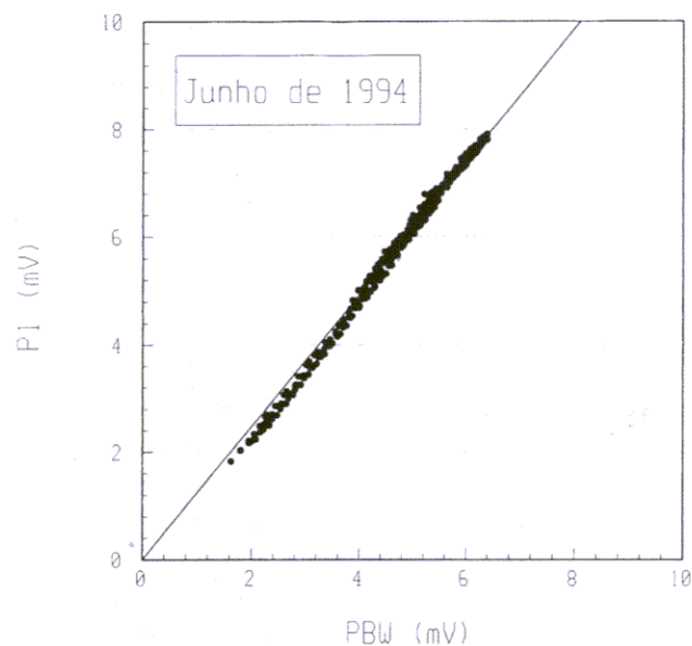
Figura 8 - Comparação entre os piranômetros protótipo P1 e de referência PBW. Valores médios de irradiância solar global calculados em intervalos de 5 minutos e observados no período de 26 a 30 de junho de 1994, na cidade de São Paulo. A curva contínua corresponde a reta de regressão que foi ajustada através do método dos mínimos quadrados passando pela origem.
